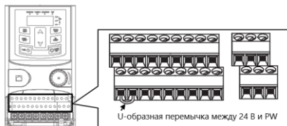
Рис. 3-7 Положение перемычки U-типа
