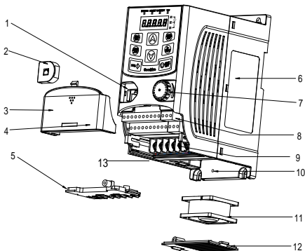
Рис. 2-2 Структурная схема ПЧ (3ф 380В, ≤4 кВт)
