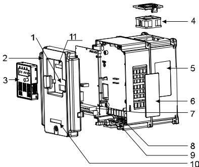
Рис. 2-3 Структурная схема ПЧ (3-ф 380 В, \geq 5.5 кВт)
